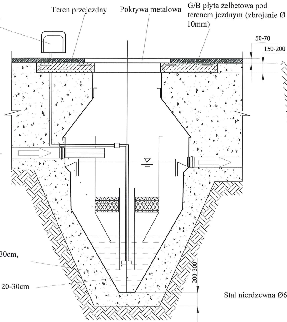
MONTAŻ OCZYSZCZALNI POD TERENEM PRZEJEZDNYM
