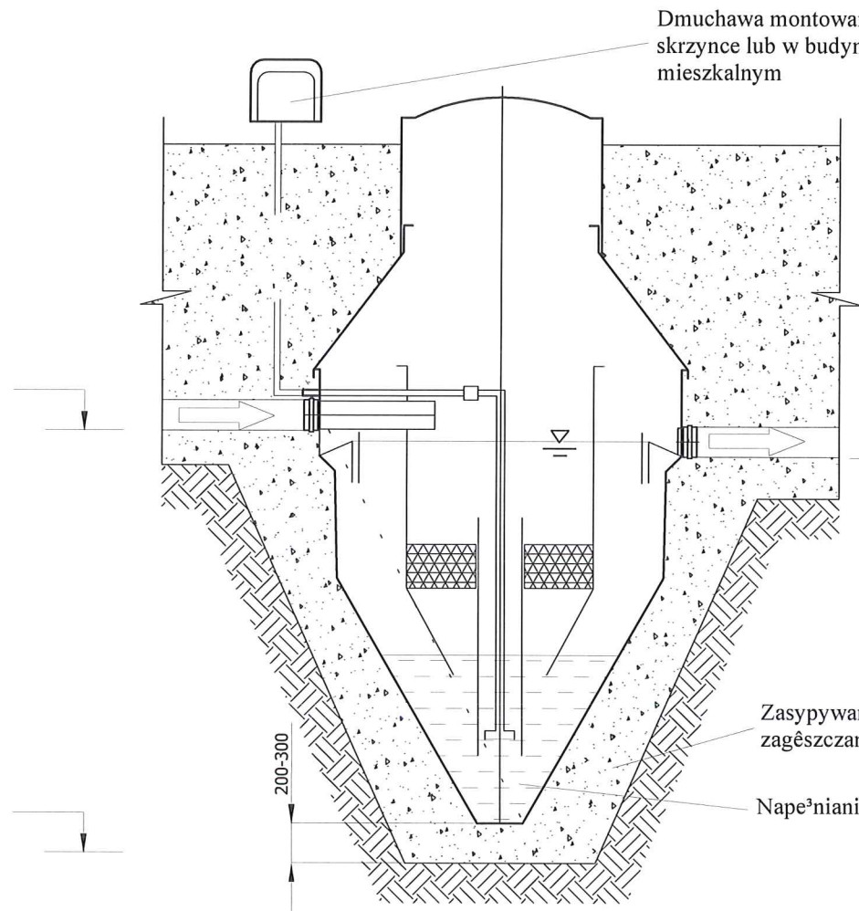
MONTAŻ OCZYSZCZALNI POD TRAWNIKIEM
